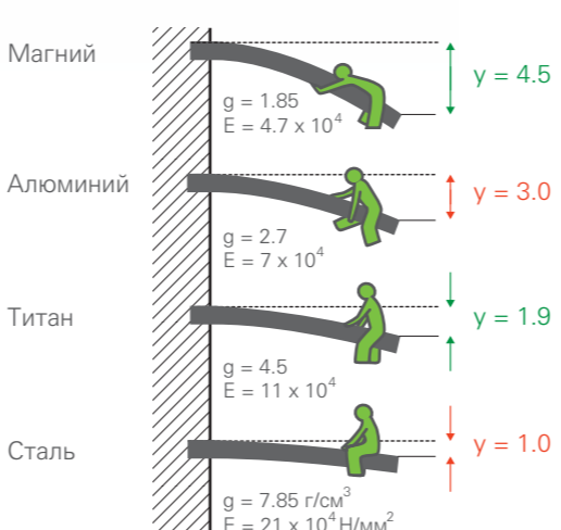
Статические характеристики
